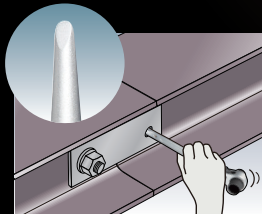
孔对准作业
